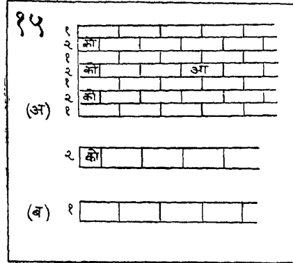
१५. Stretching bond : आडवी
